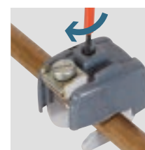
Verrouillage final par vis
