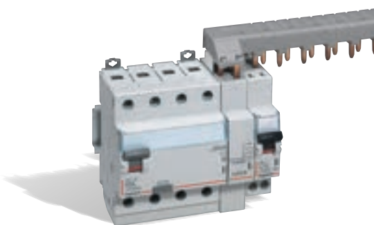
Connexion par peigne HX 3 optimisé tétrapolaire sur interrupteur différentiel DX 3
